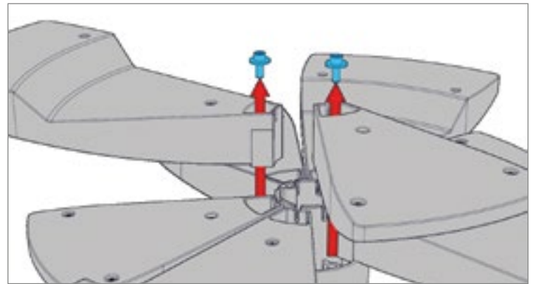
Possibilité de changer chaque pétale individuellement. Each petal can be changed independently.
